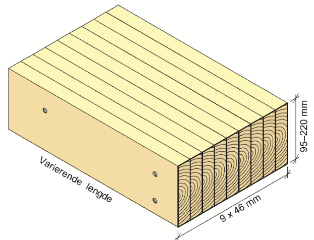
Fig. 2 Oppbygning av kantstilt element
