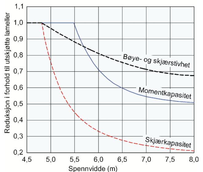
Fig 3 Reduksjon av tverrsnittsverdier til Norsk Massivtre gitt i tabell 2 for elementer med spennvidder større 4,8 m.
