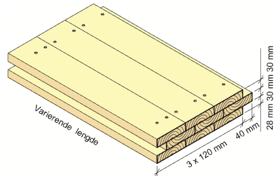
Fig. 1 Oppbygning av overlappende elementer
